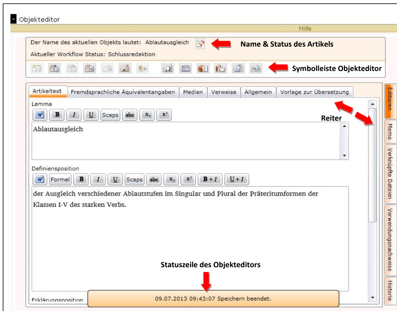
Abbildung 2: Objekteditor Artikel
